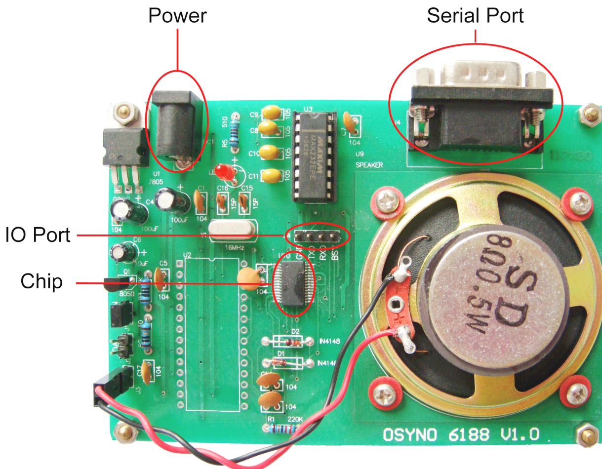
OSYNO 6188 评估板平面示图
