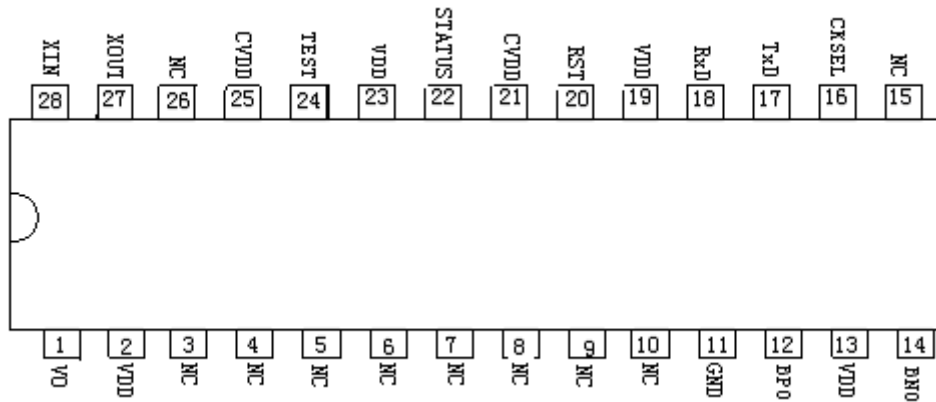
图表2 引脚结构图
